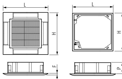
Unità interna / Indoor unit
