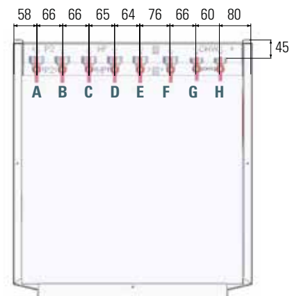
Vista superiore predisposizione attacchi idraulici Top view predisposition of hydraulic connections
