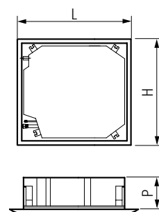
Unità interna / Indoor unit
