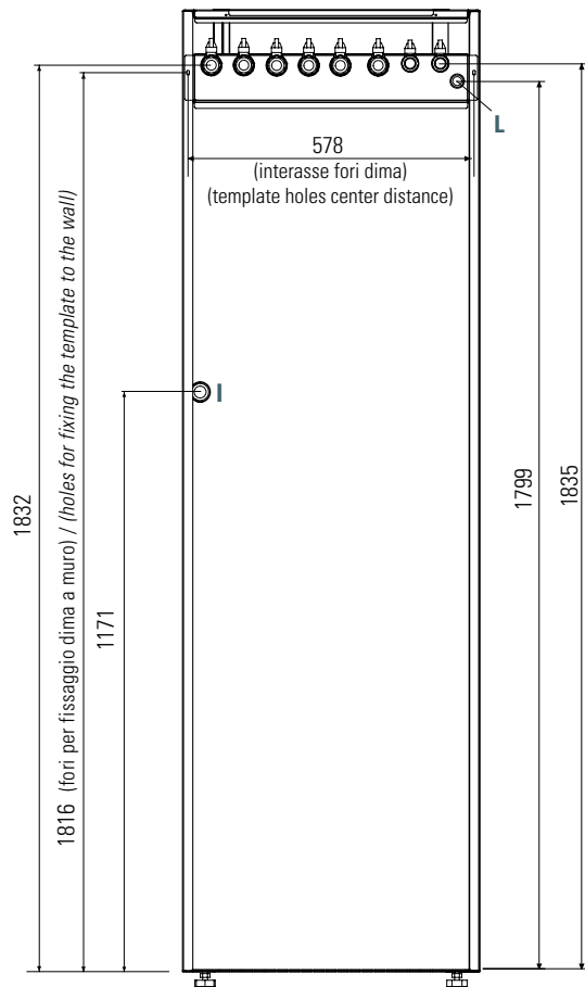
Vista frontale predisposizione attacchi idraulici Frontal view predisposition of hydraulic connections
