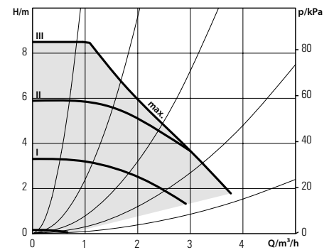
Velocità costante / constant speed I, II, III
