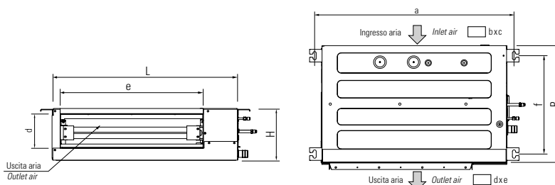
Unità interna / Indoor unit
